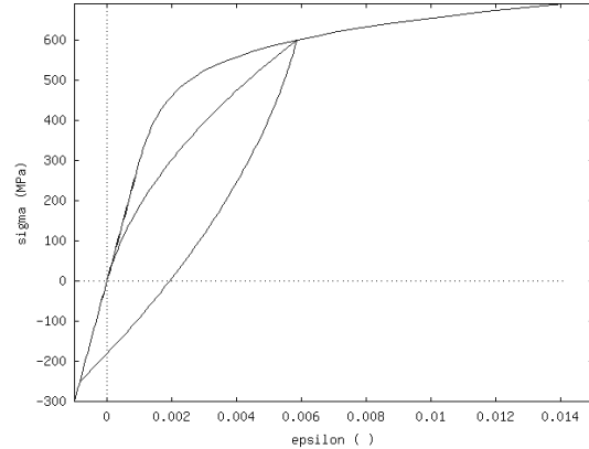
Fig. 5(b). Courbe contrainte-déformation, cas de la traction-compression.
