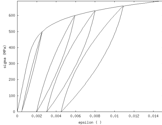
Fig. 5(a). Courbe contrainte-déformation, cas des charges-décharges.
