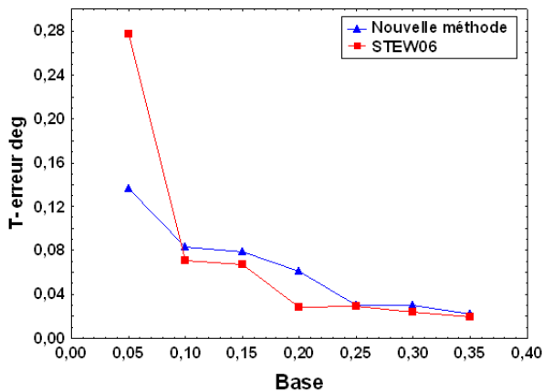
Figure 10. Erreurs sur l'orientation de la base, avec la base selon X et un objet non plan, pour des valeurs de base allant jusqu'à 0.35. On note que le nouvel algorithme fonctionne de façon satisfaisante, avec des résultats très proches de ceux de Stewenius.
