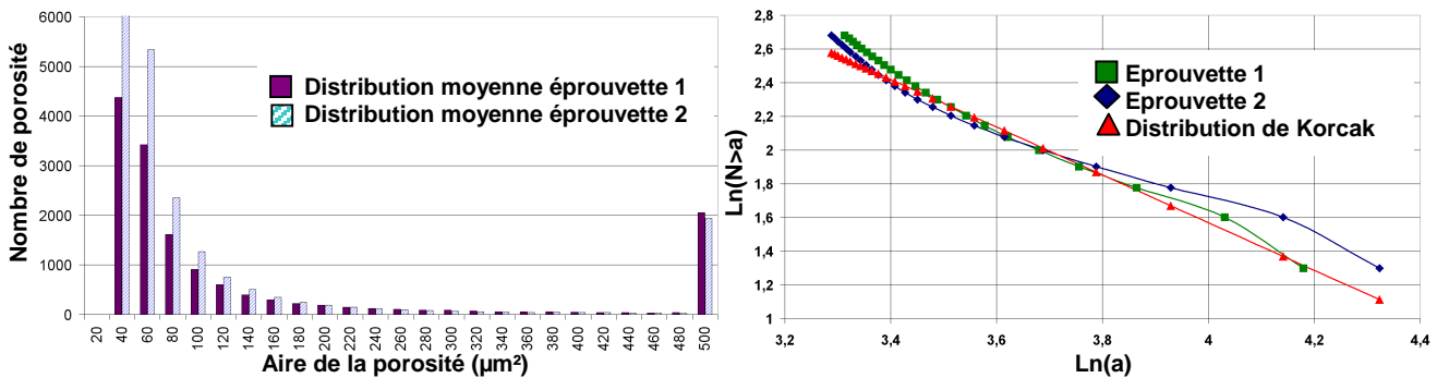
Fig. 5. Distribution granulométrique.
