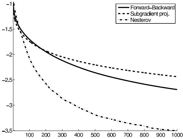
FIG. 2 – Décroissance avec k de l'erreur \log_{10}(\|f^{(k)} - f^*\|/\|f^*\|) pour l'algorithme dual avec itération explicite-implicite (trait plein), avec itérations de Nesterov (trait plein-pointillés) et par projection de sous-gradient [4] (trait en pointillés), avec \tau = \|f_0\|_{TV}/4 .
