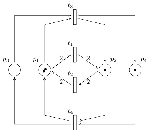
Fig. 1. Petri net.
