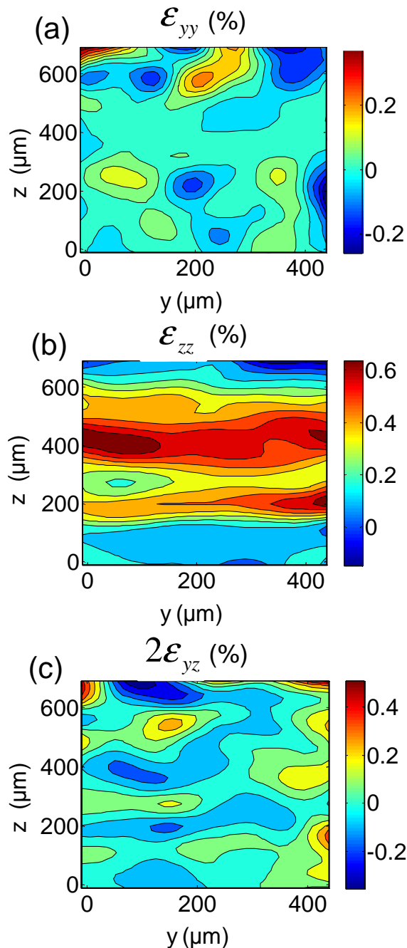
Figure 5 : (a) Carte de la déformation \epsilon_{yy} , (b) carte de la déformation \epsilon_{zz} et (c) carte de la déformation de cisaillement 2\epsilon_{yz} dans le plan (\mathbf{e}_y, \mathbf{e}_z) .
