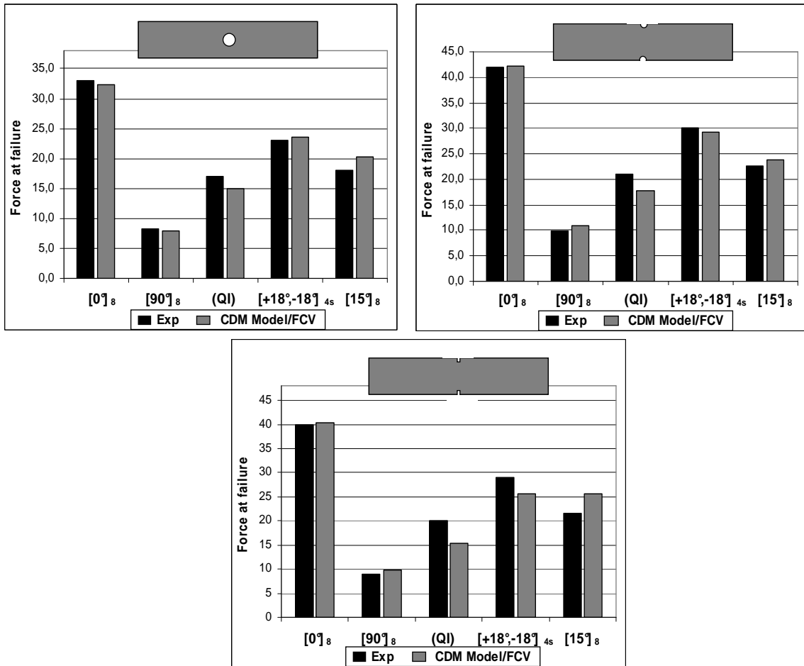
Figure 3 - Comparaison entre essais et simulations numériques pour divers stratifiés : [0], [90], [QI], [ \pm 18 ], [15]
