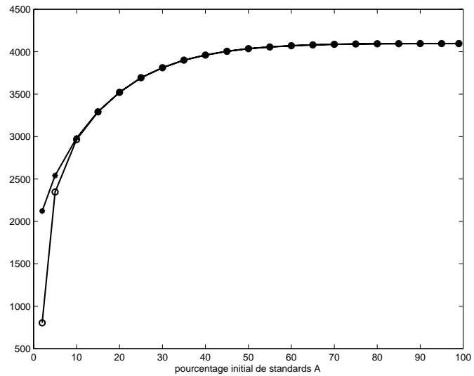
FIG. 10 – Taille de la plus grande composante connexe pour le champ (C) et le champ (C_0) correspondant dans le cas de la règle d’Ising avec \beta = 1 . (C) : * ; (C_0) : \circ
