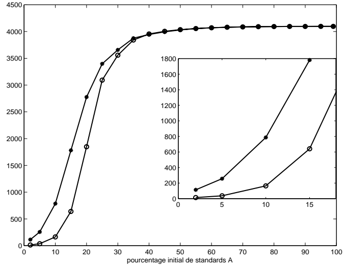
FIG. 9 – Taille moyenne des composantes connexes pour la règle d’Ising avec \beta = 1 pour les champs (C) et (C_0) correspondants. (C) : * ; (C_0) : \circ
