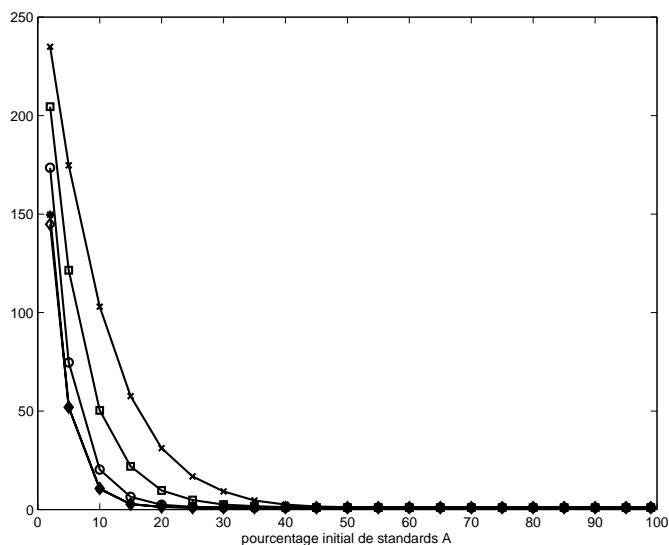
FIG. 8 – Nombre moyen de composantes connexes pour les champs ( C_0 ) associés aux champs (C) : x : faible ; □ : Ising \beta = 0.5 ; o : Ising \beta = 1 ; ◇* : Ising \beta = 3 et forte (distinctes pour la plus petite valeur de \tau )
