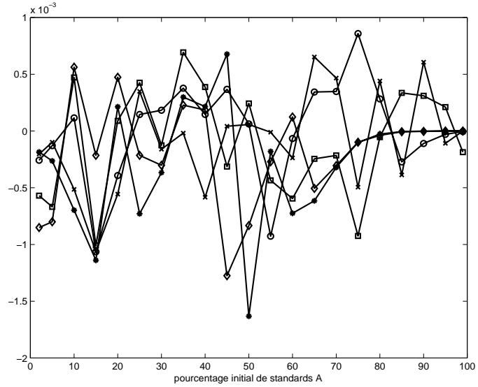
FIG. 4 – Corrélation à distance 1 pour les champs ( C_0 ) correspondant aux champs ( C ) : x : faible ; □ : Ising \beta = 0.5 ; o : Ising \beta = 1 ; ◇ : Ising \beta = 3 ; * : forte
