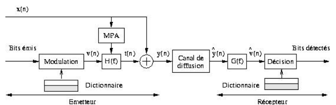
Fig. 10. Schéma de principe du système de tatouage audio.
