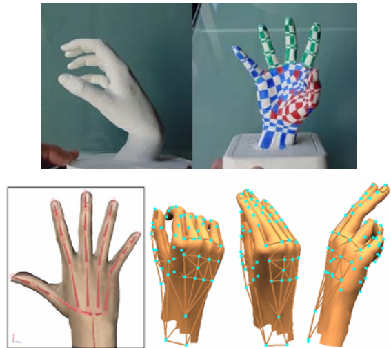
Fig. 11. En haut : Moulage de la main de la codeuse et définition du maillage de référence. En bas : Ossature, résultat après « skinning » et contrôle par le modèle de forme construit à partir des données de capture de mouvement.
