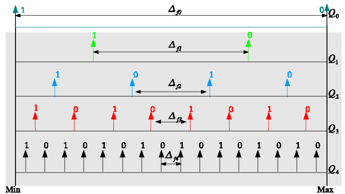
Fig. 9. Grille de quantification fractale permettant d'assurer une robustesse face aux transformations géométriques en tatouage vidéo [7].
