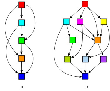
Fig. 3. a. a linear DAG. b. a non-linear DAG
