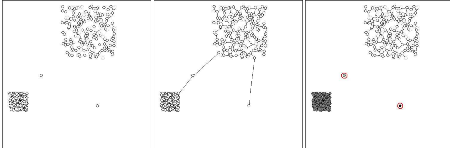
FIG. 2 – Résultats sur une base artificielle de 402 individus : 2 amas et 2 outliers.
