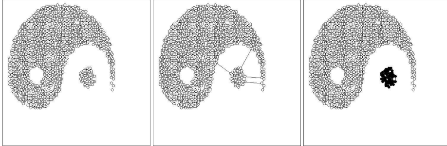
FIG. 1 – Résultats sur les données Yin et Yang.
