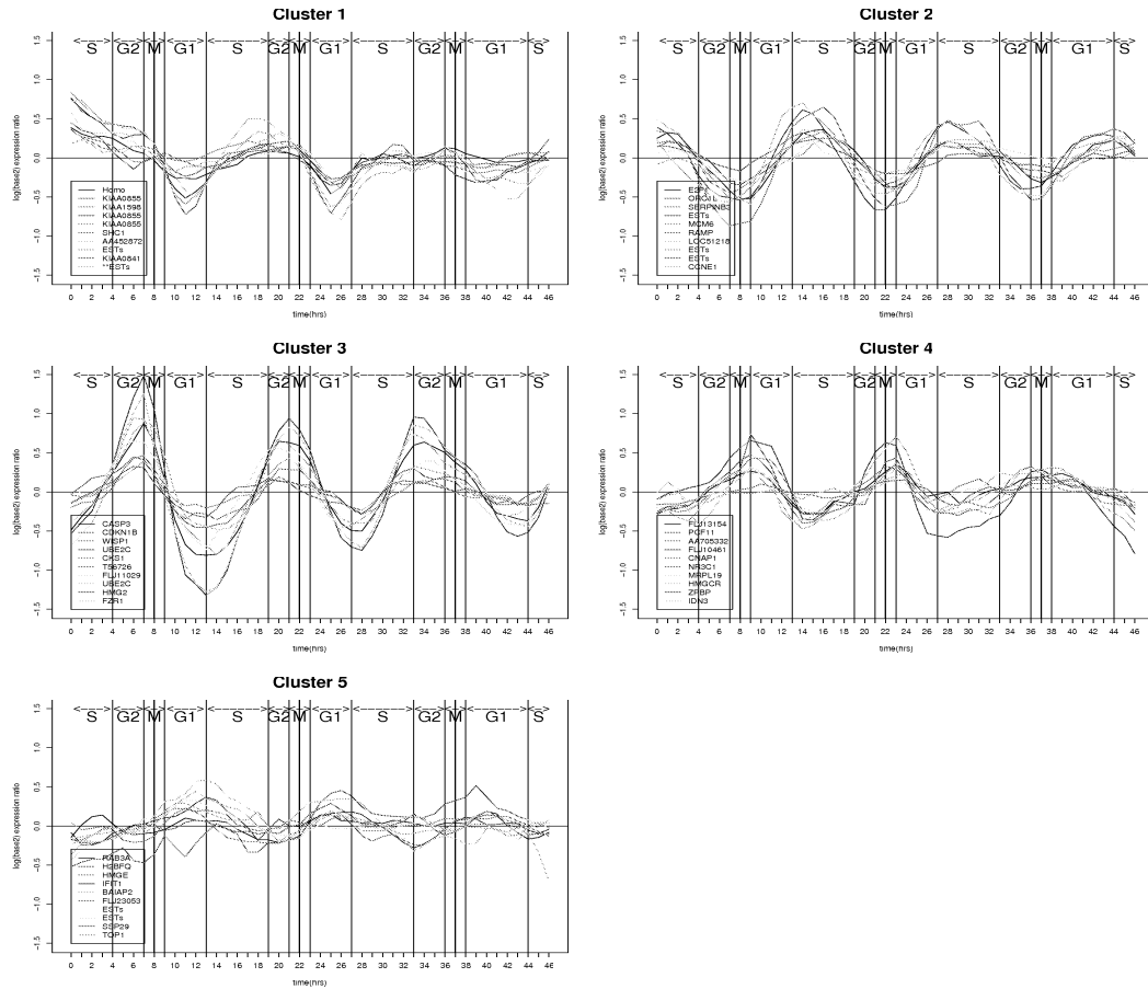
FIG. 5 – Les profils d’expression des gènes noyau durant le cycle de la division cellulaire.
