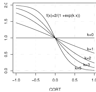
FIG. 2 – L'effet du réglage en fonction de k .
