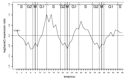
FIG. 1 – Profil d'expression du gène CCNE1 observé sur une période de 46 heures après synchronisation correspondant à trois cycles cellulaires. Les traits verticaux gras représentent les mitoses des trois cycles. Chaque phase de cycle est délimitée par les traits verticaux et annotée par G_1 , S , G_2 ou M .
