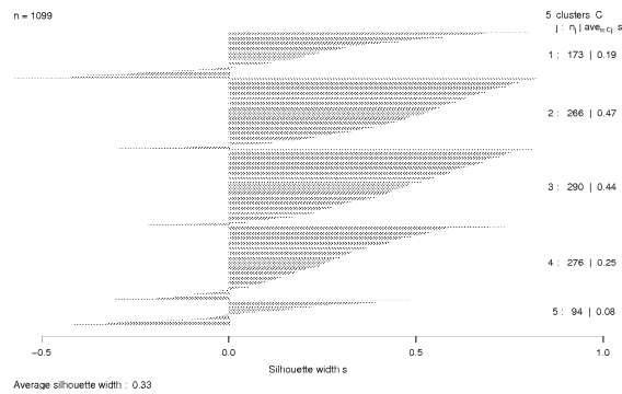
FIG. 4 – Graphe de la silhouette de P_{k^*=5.9}
