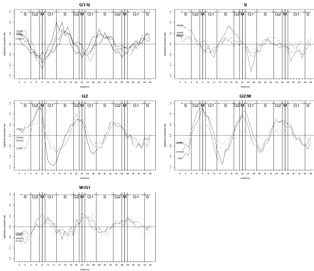
FIG. 3 – Profils des 20 gènes de référence de Whitfield et al. dont les expressions culminent dans chacune des phases suivantes du cycle cellulaire : G_1/S , S, G_2 , G_2/M et M/G_1 .
