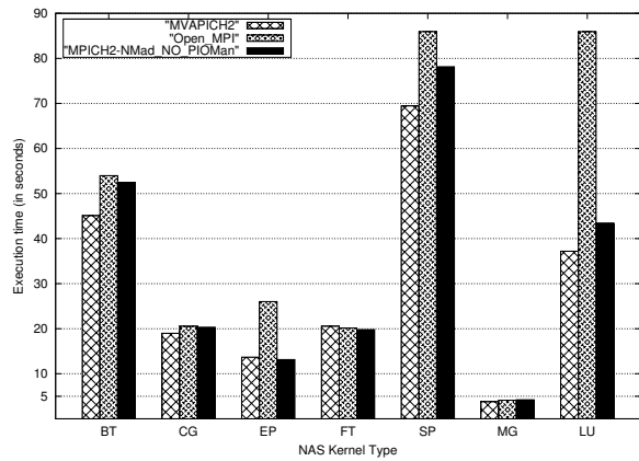
(d) 64 Processes
