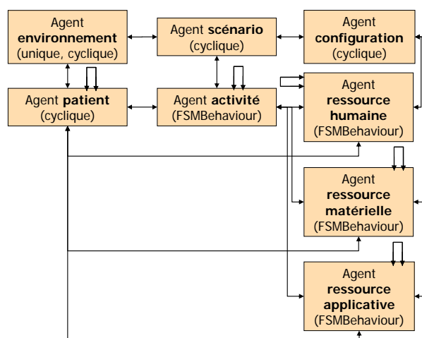
Figure 5. Architecture agents du simulateur
