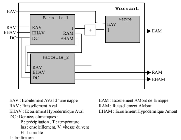
Figure 6. Modèle structurel d'un versant composé de deux parcelles, (Parcelle_1 dominante Parcelle_2)
