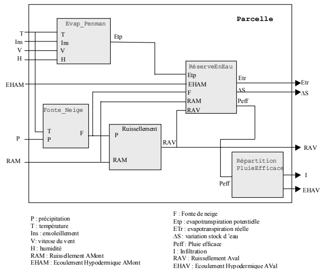
Figure 5. Modèle structurel d'une parcelle
