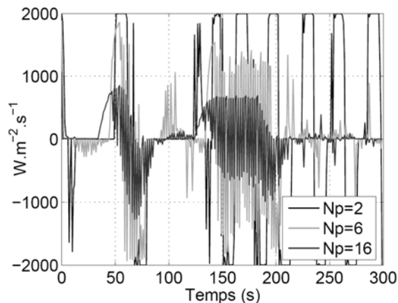
Figure 7 : Calage de l'horizon de prédiction, vitesse de variation de la commande
