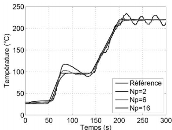
Figure 5 : Calage de l'horizon de prédiction, variable de sortie Température mesurée
