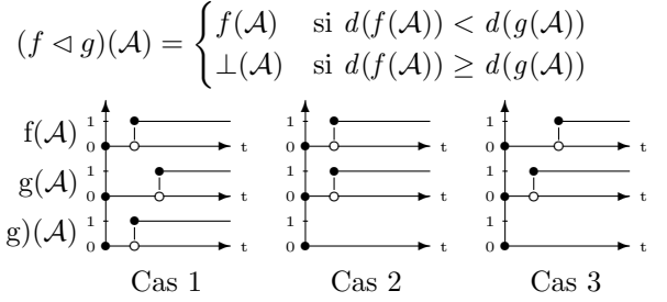
Fig. 3. Comportement attendu pour (f \triangleleft g)(\mathcal{A})
