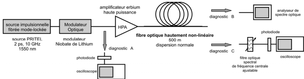
Figure 2. Dispositif expérimental.
