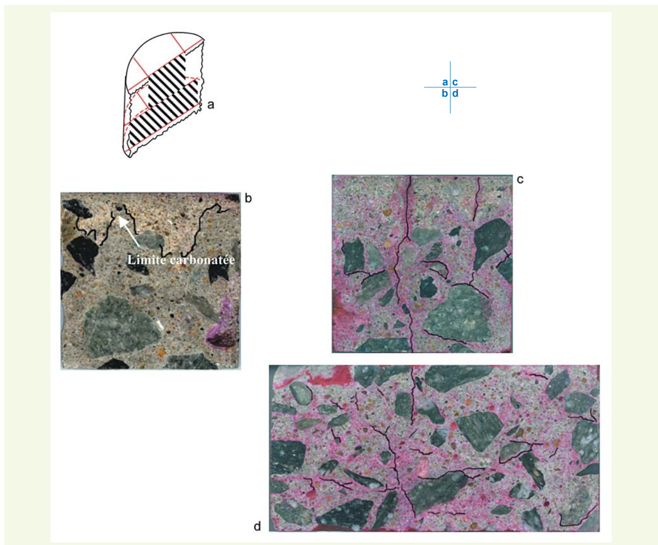
figure 4 Observation au colorant rouge des microfissures de l'éprouvette 8-2A : a : principe de sciage (avec face avant sciée), b : photo après sciage (avec tracé de la limite carbonatée, zone non carbonatée en gris foncé correspondant à la thymolphtaléine décolorée à la lumière), c et d : photos après préparation au colorant rouge (avec tracé des fissures les plus évidentes).
