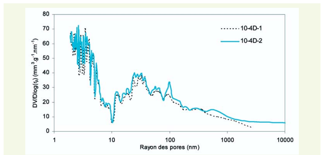
figure 1 Distribution volumique des pores à cœur dans la carotte 10-4 - Étude de répétabilité.
