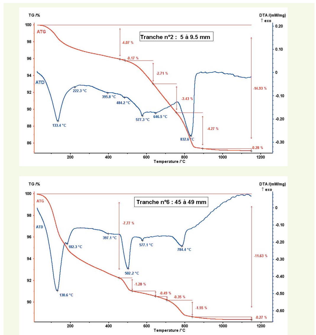
figure 5 Courbes ATG/ATD de l'éprouvette 8-8A tranches 2 et 6 (ATG : analyse thermogravimétrique ; ATD : analyse thermique différentielle).
