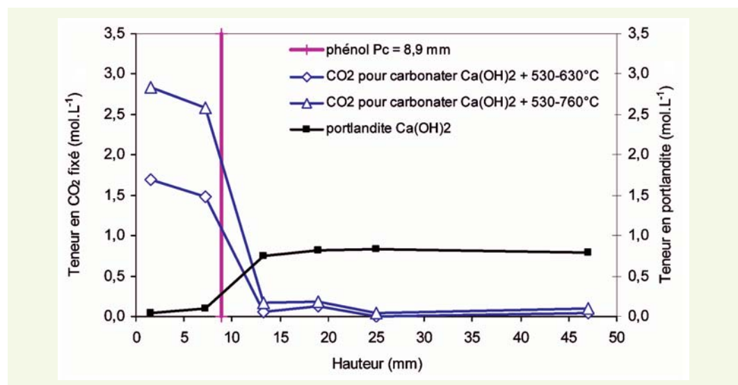
figure 6 Profil de portlandite résiduelle et encadrement du profil de carbonatation de l'éprouvette 8-8A, mesuré par ATG-AC.
