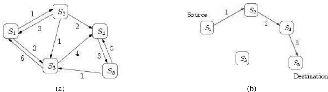
Figure 1 : Illustration d'un graphe orienté pondéré (a) et de la route optimale obtenue par parcours de ce graphe (b)
