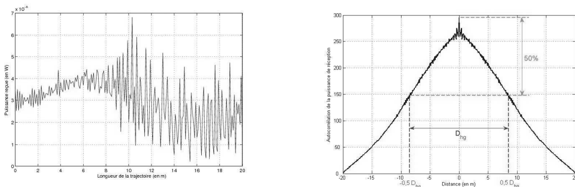
Figure 3 : Illustration de l'évolution de la puissance reçue pour une trajectoire et de la fonction d'autocorrélation associée
