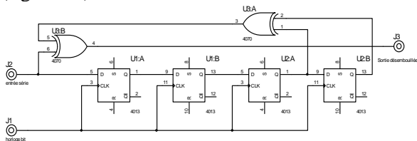
Fig 10 : Descrambler
