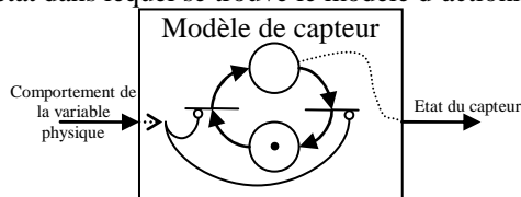
Figure 10. Modélisation d'un capteur par un réseau de Petri
