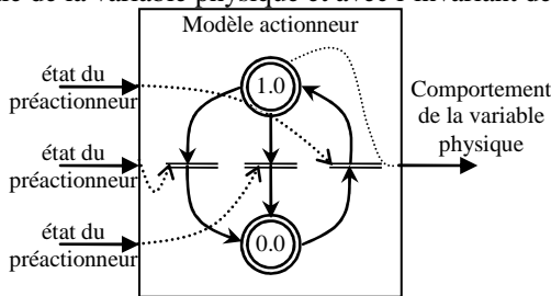
Figure 9. Modélisation de l'actionneur par un réseau de Petri continu
