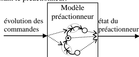
Figure 8. Modélisation du préactionneur par un réseau de Petri discret
