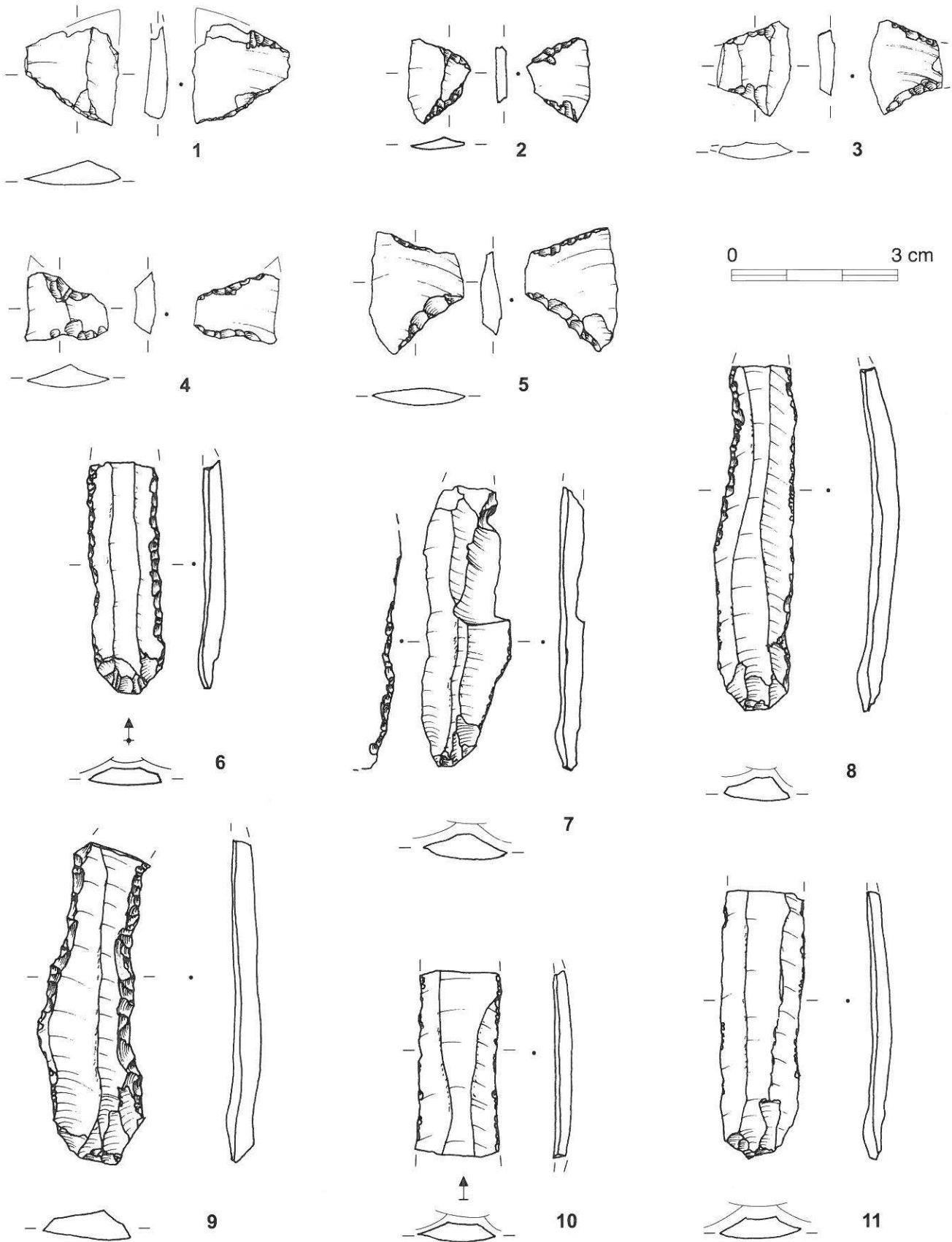
Fig. 8 : Quelques éléments de l'industrie lithique de l'horizon épicald (dessins T. Perrin).
