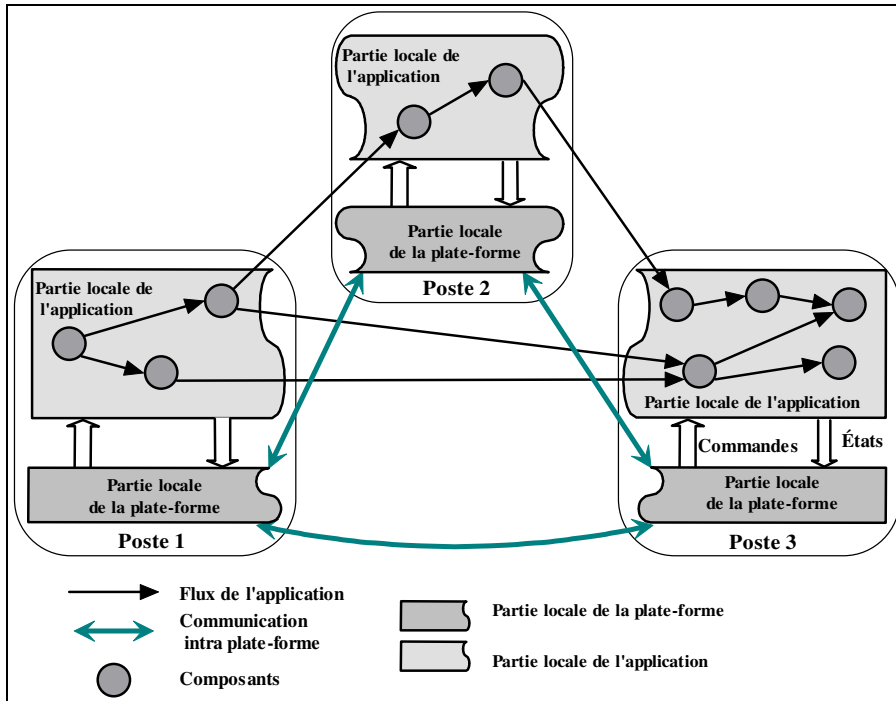
Figure 4. Supervision de l'application par la plate-forme Kalinahia
