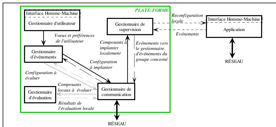
Figure 9. Structure de la plate-forme Kalinahia
