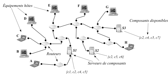
FIG. 1 – Illustration du déploiement de composants dans un réseau d’infrastructure
