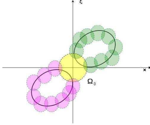
Fig. 5 : Ouvert \Omega_0 où la forme normale est valide.
