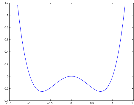
Fig. 3 : La courbe représentative de la fonction potentiel paire V(x) = x^4 - x^2 . On distingue les deux puits (les minima) du potentiel, le droit et le gauche.
