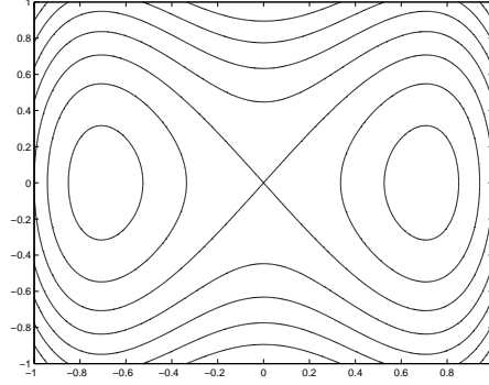
Fig. 4 : Le feuilletage de p^{-1}(c) ; avec des c > 0 les fibres elliptiques ont une seule composante connexe, pour c=0 : la fibre singulière en forme de huit hyperbolique, et pour des c < 0 : les fibres elliptiques ont deux composantes connexes.
