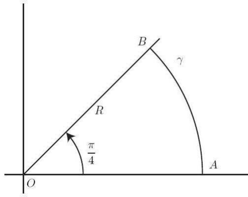
Fig. 9 : Chemin d'intégration \gamma_{\epsilon,R} := L_{\epsilon,R} \cup C_R \cup [R, \epsilon] \cup C_\epsilon .
