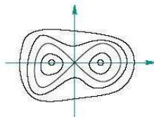
Fig. 1 : Le feuilletage autour d'une singularité hyperbolique dans l'espace de phases.
