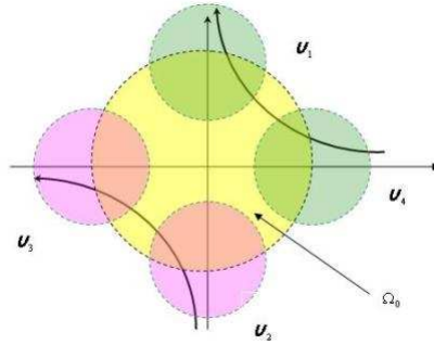
Fig. 6 : Les ouverts U_1, U_2, U_3, U_4 et \Omega_0 .
