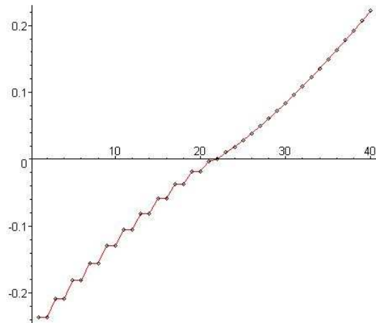
Fig. 7 : Tracé numérique d'une partie du spectre du double puits symétrique : sur l'axe des abscisses on trouve un indexage des valeurs propres, et sur l'axe des ordonnées on trouve les valeurs propres.
