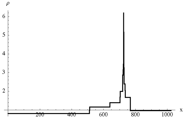
Fig. 24a. The Turcotte cascade for (de Wijs parameters d=0.2 hence \mu\epsilon_+=1.2 hence \gamma_+=0.27 ).
