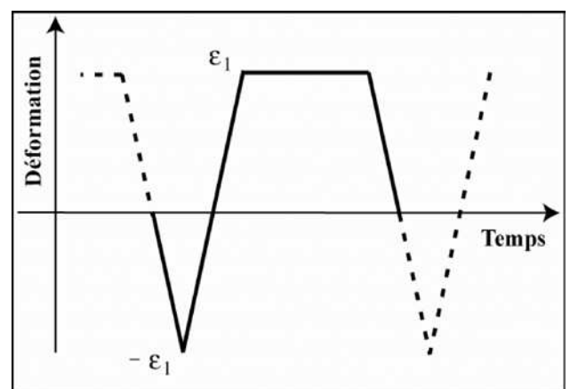
Fig. 1 - Principe d'un essai d'érouissage cyclique.
