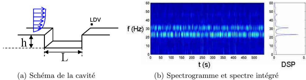
Fig.1. Schéma de l'expérience et spectrogramme du signal LDV. Dans le cas étudié, U = 2,09 \text{ m.s}^{-1} , deux pics à f_1 = 23.2 \text{ Hz} et f_2 = 31.0 \text{ Hz} apparaissent clairement dans le spectre.
