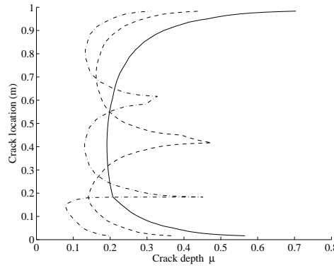
(d) \mu = 0.2 and L_{crack} = 0.55m
