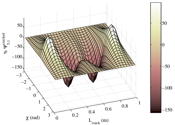
(d) \% \Psi_{5,1}^{cracked} for \mu = 1
