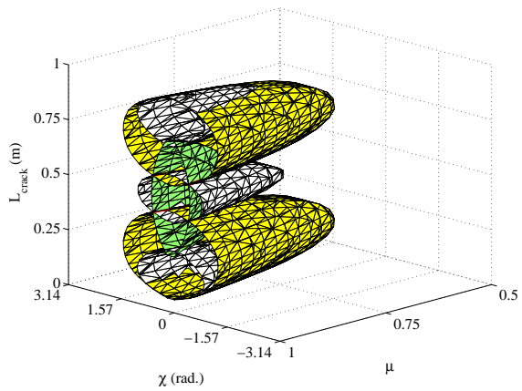
(d) \mu = 0.9, \chi = \frac{\pi}{10}rad., L_{crack} = 0.42m
