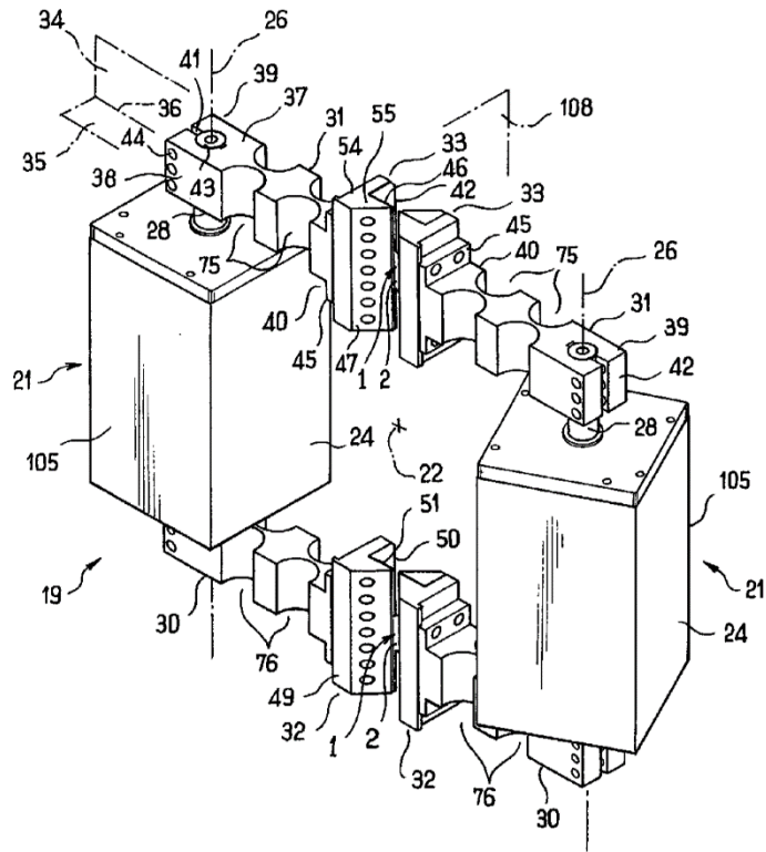
Figure de principe du dispositif. Brevet n° EP1530709 (A2), auteurs : Sylvain Calloch, David Dureisseix, Gilles Arnold, Inaki Zudaire Rovira.
