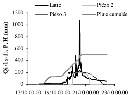
Fig. 5 Crue du 20 octobre 2001 sur le bassin versant de la Latte. Qi : débit instantané. P : précipitations. H : hauteur d'eau dans les piézographes.
