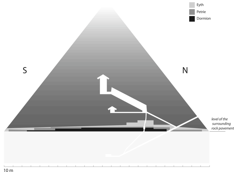
Figure 17. Kheops Pyramid NS cross section showing the earlier data on the original hill morphology. Figure 17. Pyramide de Kheops. Section NS montrant les données antérieures sur la géométrie de la colline originelle.
