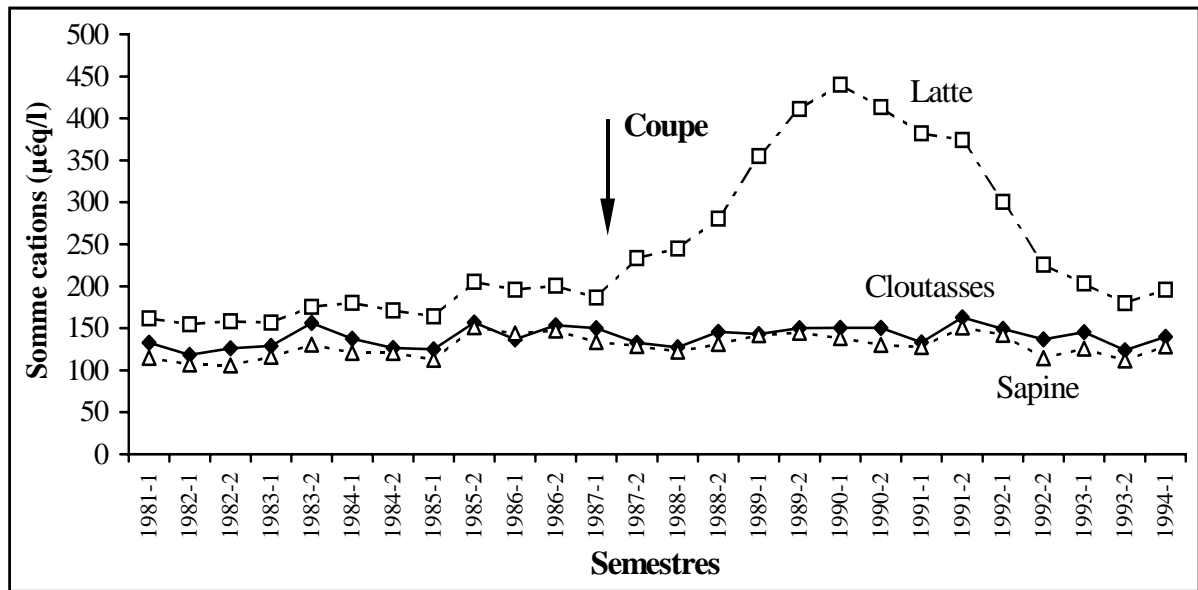
Figure 2 - Valeurs moyennes semestrielles de la somme des cations basiques ( \mu\text{eq./l} ) dans les eaux des ruisseaux des Cloutasses, de la Latte et de la Sapine.
