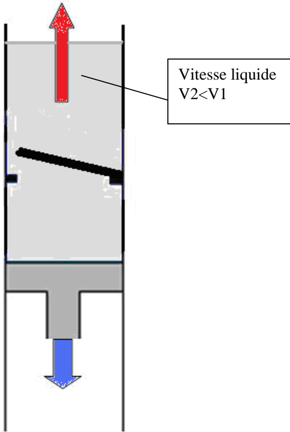
Figure A 2 : le piston continue à descendre et le liquide continue à monter avec une vitesse V_2 plus faible ( V_2 < V_1 ). Le piston continue à descendre, le clapet est entrouvert.
