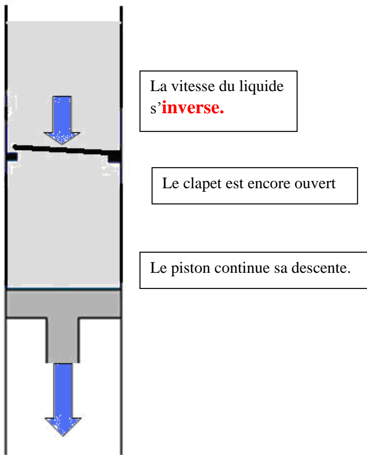
Figure A 3 : le piston descend et la vitesse du liquide s'inverse .
