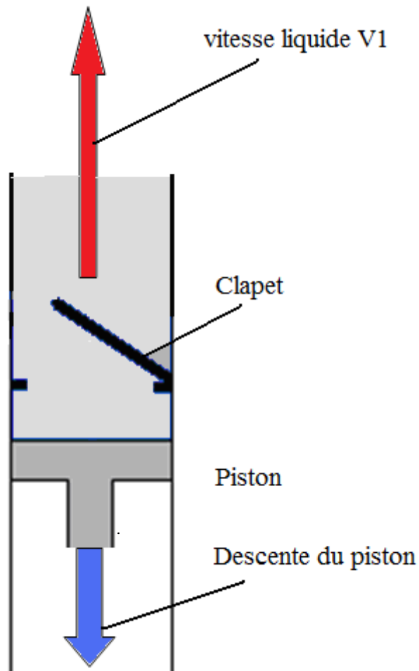
Figure A 1 : Le piston commence à descendre, le liquide continue son ascension.
