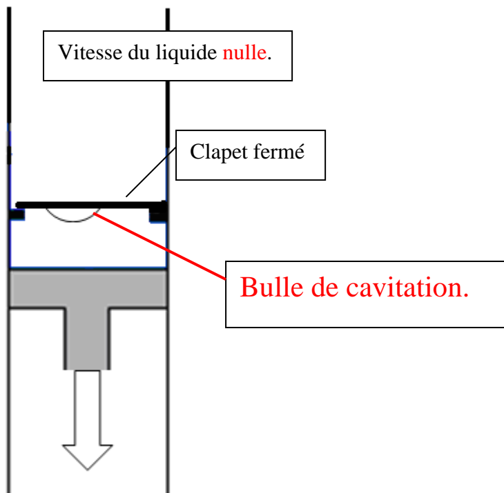
Figure 4 : le clapet se ferme brutalement avec un retard et une bulle de cavitation apparait.
