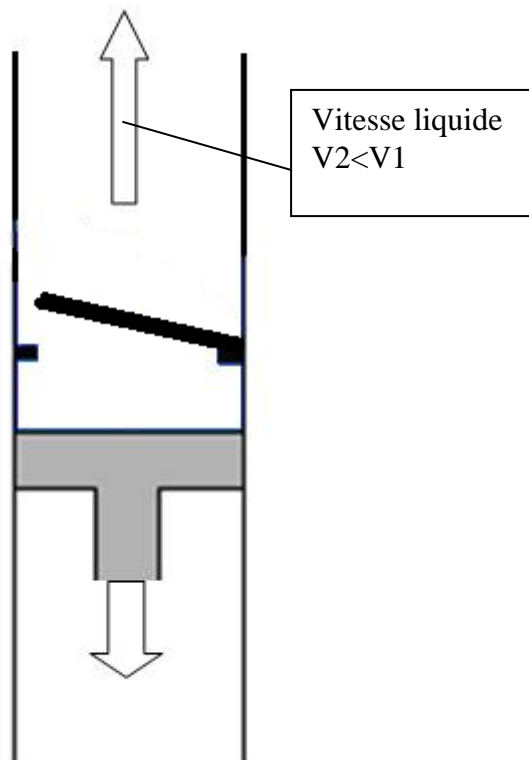
Figure A 2 : le piston continue à descendre et le liquide continue à monter avec une vitesse V_2 plus faible ( V_2 < V_1 ). Le piston continue à descendre, le clapet est entrouvert.
