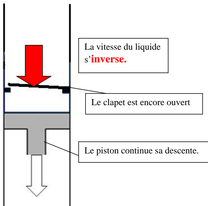
Figure A 3 : le piston descend et la vitesse du liquide s'inverse .
