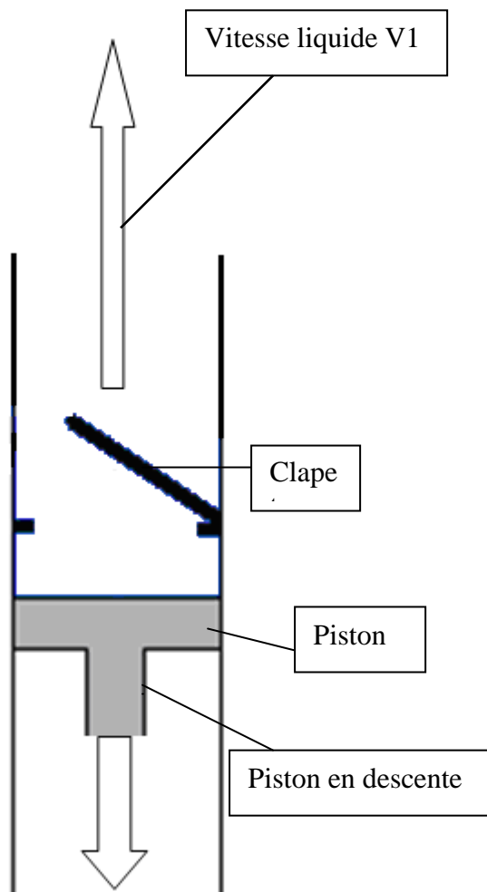
Figure A 1 : Le piston commence à descendre, le liquide continue son ascension.
