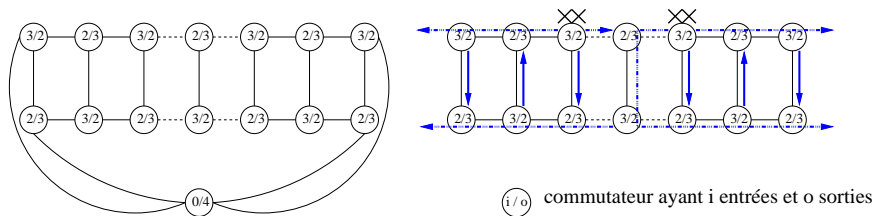
FIG. 5: Réseaux construits avec des commutateurs de degré 8 ( r = 4 ) tolérant 4 pannes et un exemple de routage pour un jeu de 4 pannes.
