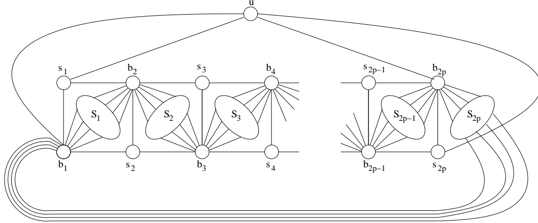
FIG. 6: Réseaux construits avec des commutateurs de degré 2r pour r > 4 et tolérant 4 pannes.
