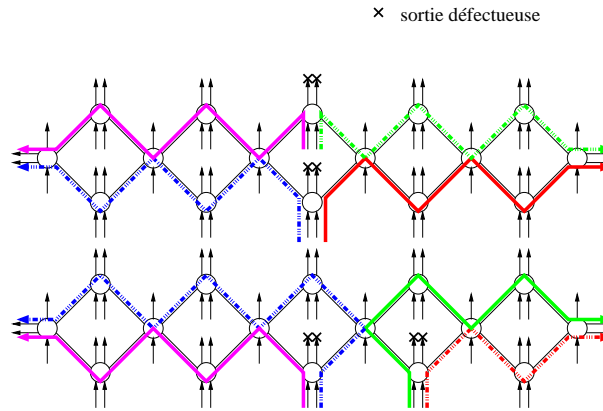
FIG. 4: Les entrées sont routées localement sur les sorties attenantes lorsqu'elles sont valides. Les 4 entrées qui ont perdu leurs sorties locales utilisent les chemins arêtes-disjoints représentés sur la figure pour atteindre des sorties valides.
