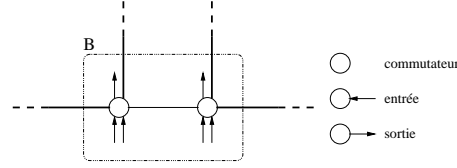
FIG. 1: Exemple de bloc pour r = 3 . Il vérifie : \delta(B) = i(B) + 2 - o(B) = 4
