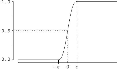
FIGURE 14. Function H_\varepsilon .
