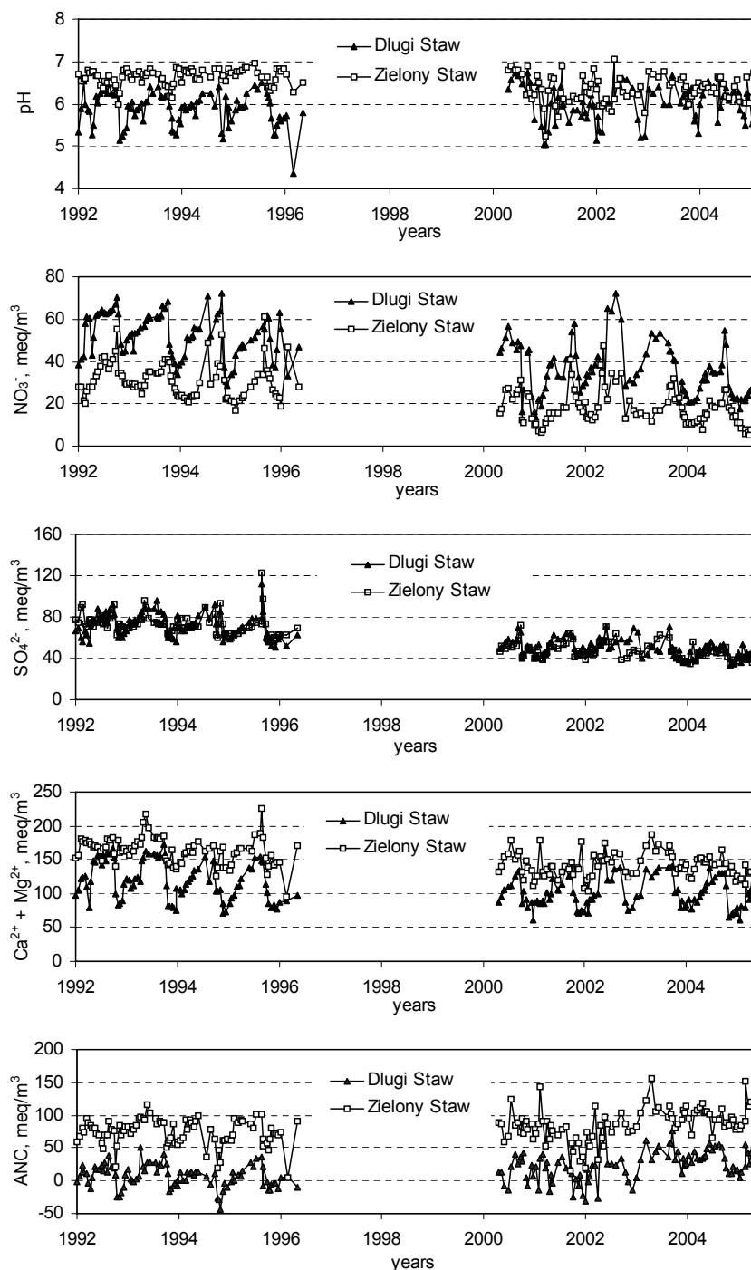
Fig. 6. Major chemical parameters in lake outflow from Długi Staw and Zielony Staw.
