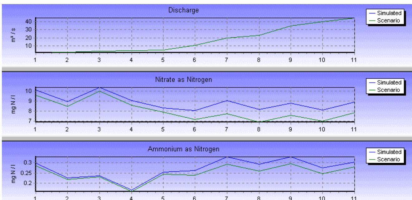
Fig. 11. Scenario 2: day 30
