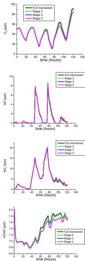
Fig. 10. Plots for PUMA trajectory run for O 3 , NO, NO 2 , HCHO.
