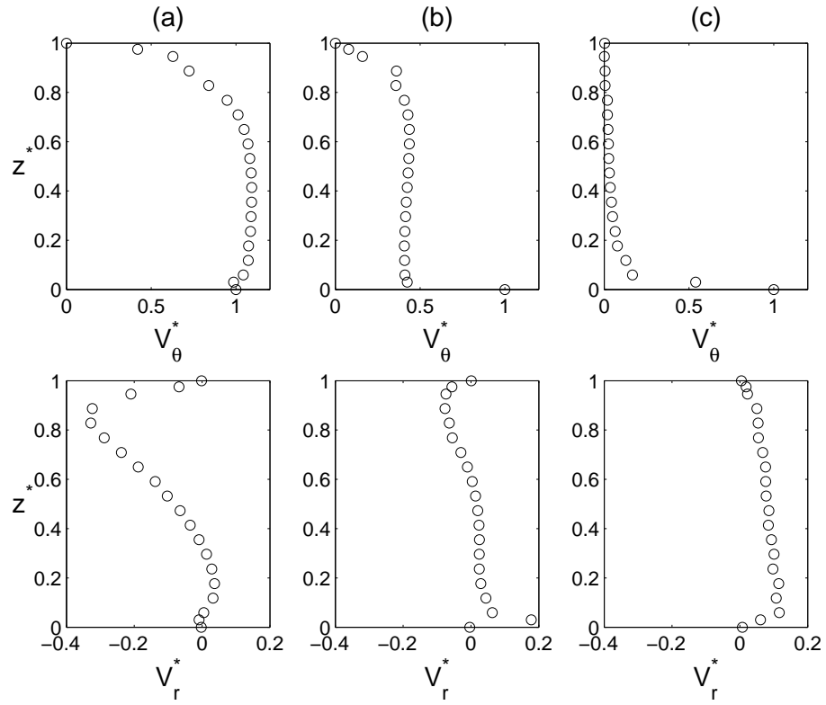
Figure 2: Profils axiaux des composantes radiale V_r^* et tangentielle V_\theta^* de la vitesse moyenne à r^* = 0.56 pour Re = 1.04 \times 10^6 , G = 0.036 et trois valeurs de C_w : (a) C_w = 5929 , (b) C_w = 0 , (c) C_w = -5929 .
