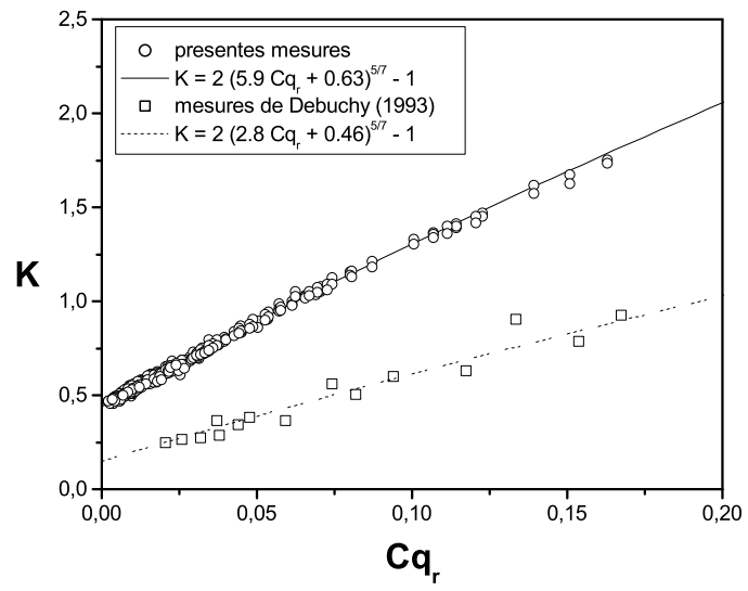
Figure 5: Influence de la prérotation sur la loi de puissance en 5/7 liant K à Cq_r .
