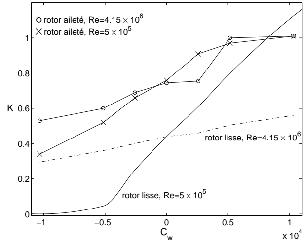
Figure 8: Évolution de K en fonction de C_w en r^* = 0.8 . Comparaison entre le cas lisse et le cas où le rotor est muni de 10 ailettes pour G = 0.036 .
