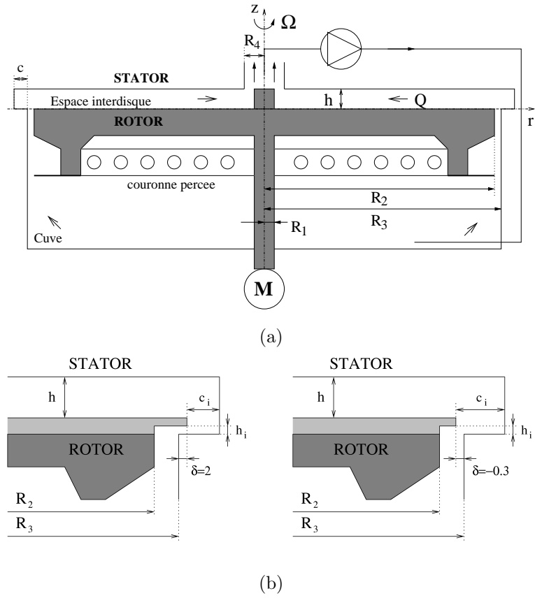
Figure 1: (a) Schéma général du dispositif interdisque avec R_1 = 38.5 , R_2 = 250 , R_3 = 253 , R_4 = 55 , 1 \leq h \leq 12 et 0 \leq c \leq 5 ; (b) Géométries considérées en périphérie de la cavité avec c_i = 3 , \delta = [-0.3; 2] et h_i variable. Toutes les longueurs sont données en mm.
