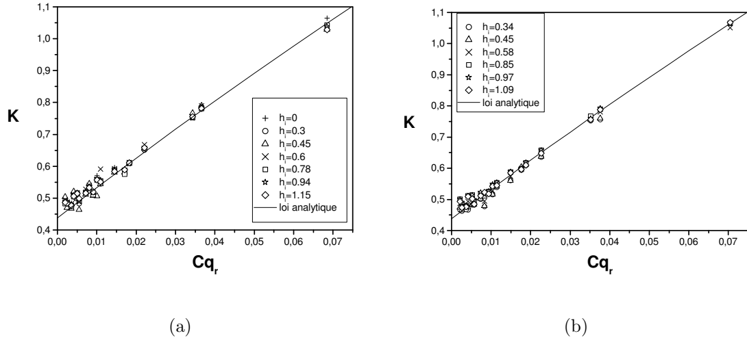
Figure 6: Influence de la géométrie en entrée de la cavité sur la loi analytique (8) pour G = 0.036 , Re = 4.15 \times 10^6 et C_w = [2579; 5159; 10317] (mesures par LDA): (a) Recouvrement négatif \delta = -0.3 mm - (b) Recouvrement positif \delta = 2 mm.
