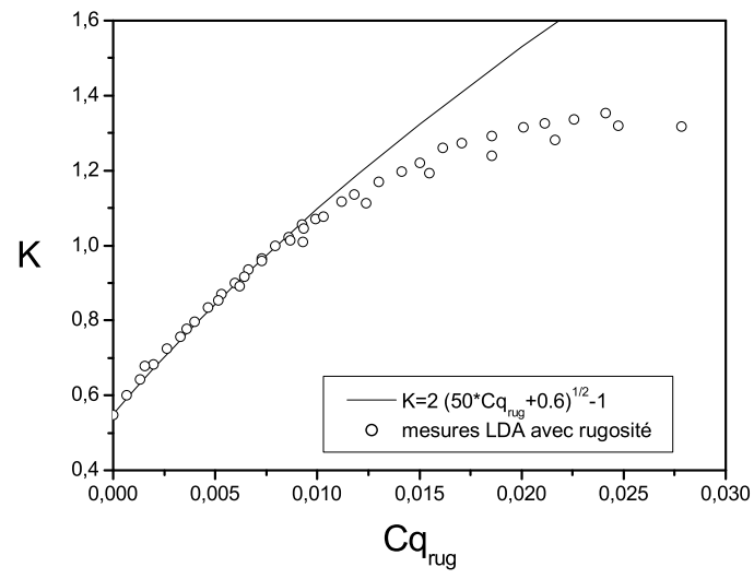
Figure 7: Loi d'évolution de K en fonction de Cq_{rug} dans la configuration rotor rugueux / stator lisse.
