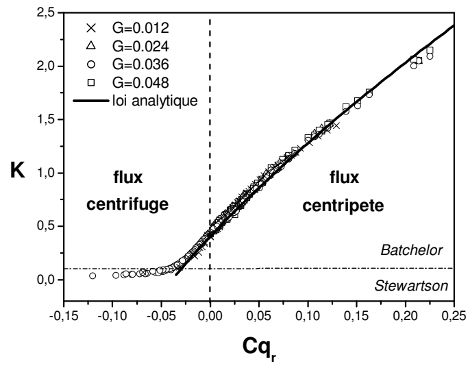
Figure 4: Loi liant K à Cq_r pour des écoulements turbulents de type Batchelor. Influence du rapport d'aspect de la cavité: ( \times ) G = 0.012 , ( \Delta ) G = 0.024 , ( \circ ) G = 0.036 , ( \square ) G = 0.048 , (—) loi analytique.
