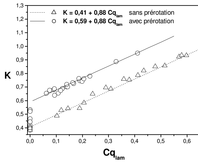
Figure 9: Loi liant K à Cq_{lam} dans le cas d'écoulements laminaires entre deux disques lisses avec ou sans prérotation.
