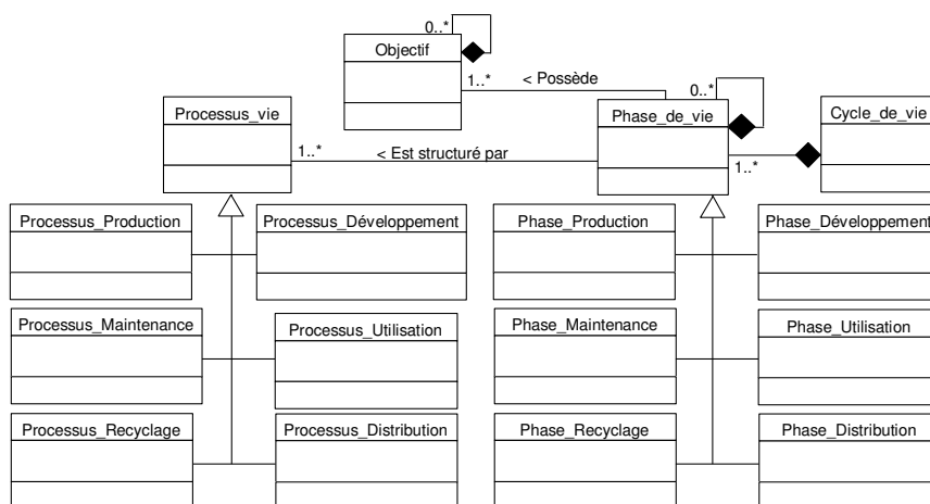
Figure 4. Modèle UML du cycle de vie
