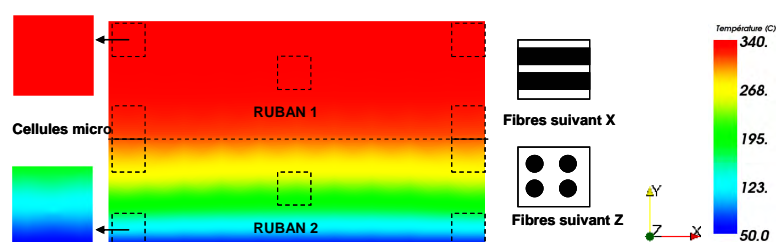
FIG. 4 – Champ de température obtenu après simulation d'un essai de refroidissement sur un composite constitué de 2 rubans de préimprégné
