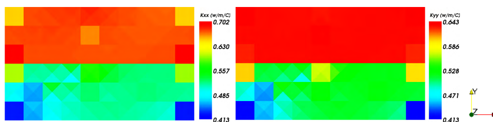
FIG. 5 – Composantes K_{xx} et K_{yy} du champ de conductivité thermique homogénéisé ( W.m^{-1}.^{\circ}C^{-1} )
