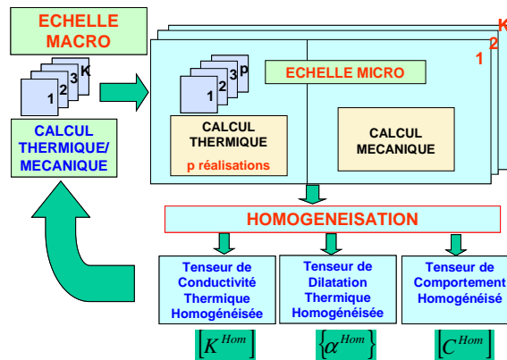
FIG. 3 – Diagramme de l'algorithme général du calcul multi-échelle
