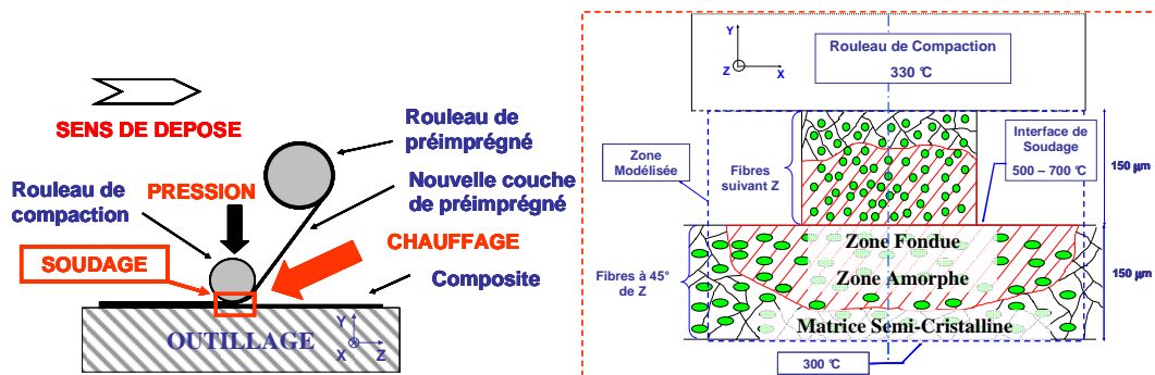
FIG. 1 – Schéma représentatif du procédé d'empilement par soudage et consolidation en continu (à gauche) et schéma représentatif des phénomènes mis en jeu au cours du procédé (à droite)
