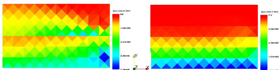
FIG. 6 – Composantes \sigma_{xx} et \sigma_{yy} du champ de contrainte (MPa) obtenu après simulation
