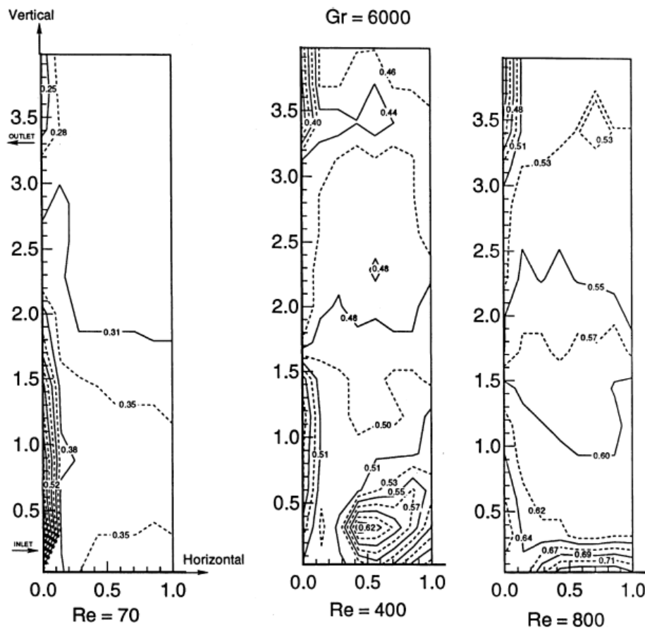
Fig. 8 : Coupes horizontales des températures pour différentes valeurs du nombre de Reynolds Re et un nombre de Grashof 2 Gr constant.
