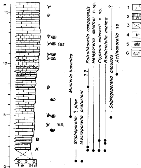
Figure 9. Coupe-type de Heteroporella deloffrei n.sp. (A : Éch. BT 98) et de Clypeina estevezii n.sp. (A : Éch. BT 98 ; B : Éch. BT 81) : localisation (à gauche), colonne lithostratigraphiques (à droite). Légende : 1- calcaires micritiques, 2- oolithes, 3- lacune d'observation, 4 structures bio-sédimentaires de type Cayeuxia , 5- oncoïdes (et ooïdes des micritiques), 6- stromatolithes.
