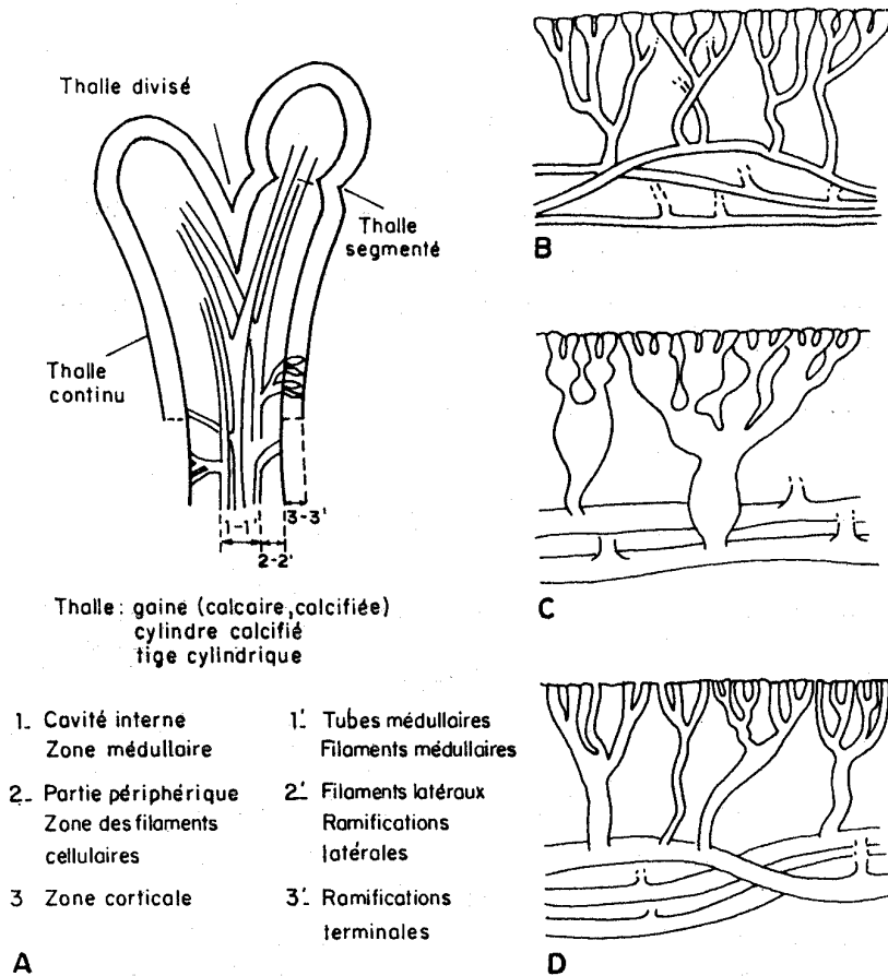
Figure 12. SIPHONALES : Représentation schématique : A d'une Udotécée (d'après J.-P. Bassoulet et alii , 1983) ; B-D des filaments médullaires et latéraux chez les genres Arabicodium (B), Halimeda (C) et Boueina (D) (d'après G.F. Elliott, 1982).
