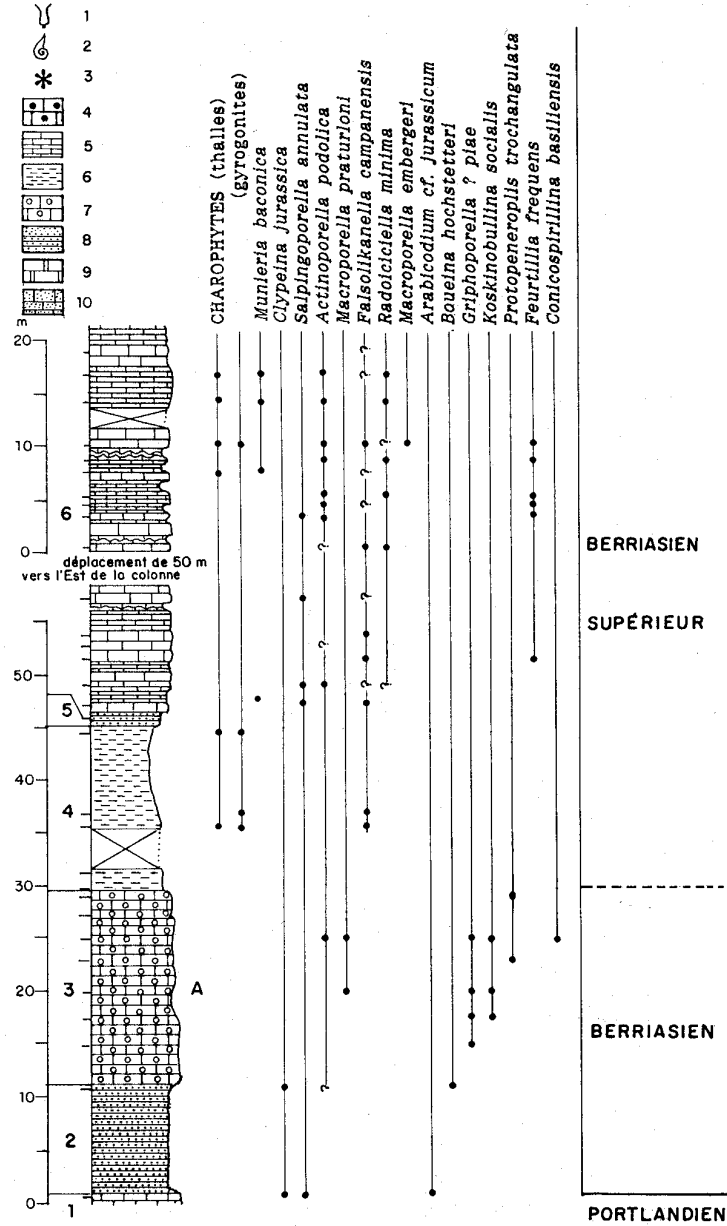
Figure 3. Puig Campana : Coupe de la Brèche de Roland. Localisation du gisement-type de Arabicodium poignantii n.sp. (A : Éch. Brèche 5). Légende : 1- Calpionelles, 2- Ammonites, 3- remaniements de matériaux triasiques, 4- calcaires à ooi des ferrugineux, 5- calcaires micritiques, 6- marnes et calcaires argileux, 7- oolithes, 8- grès et sables, 9- biolithites de Madréporaires, 10- calcarénites.
