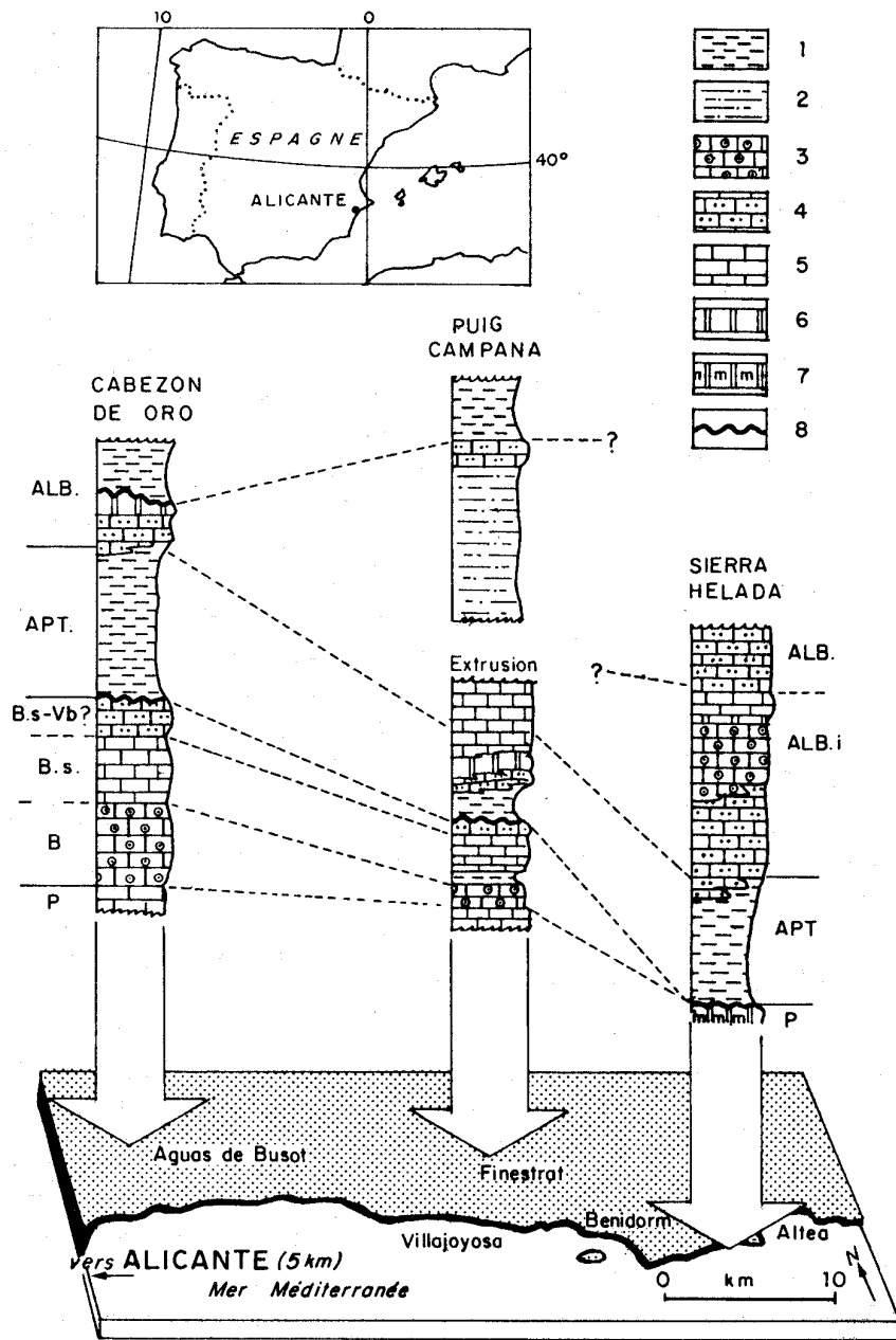
Figure 1. Jurassique terminal et du Crétacé inférieur de l'«arrière-pays de Benidorm» : Colonnes synthétiques et corrélations stratigraphiques. Légende : 1- marnes et calcaires argileux, 2- marnes et calcaires sablonneux, 3- oolithes, 4 calcarénites et grès à ciment calcaire, 5- calcaires micritiques, 6- biolithites de Madréporaires, 7- mud mounds , 8- hard grounds .
