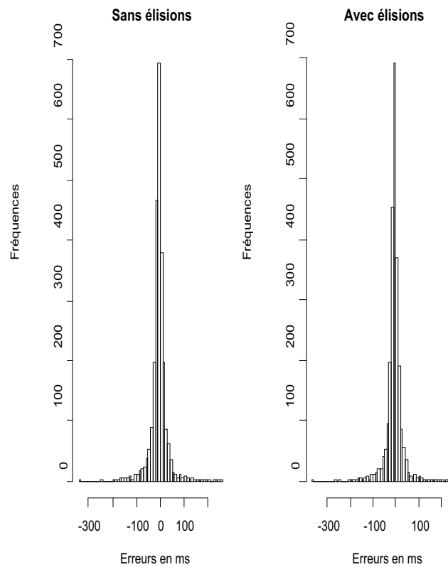
Figure 5 Histogrammes des distributions des erreurs pour les alignements fondés sur les phonétisations sans et avec élisions
