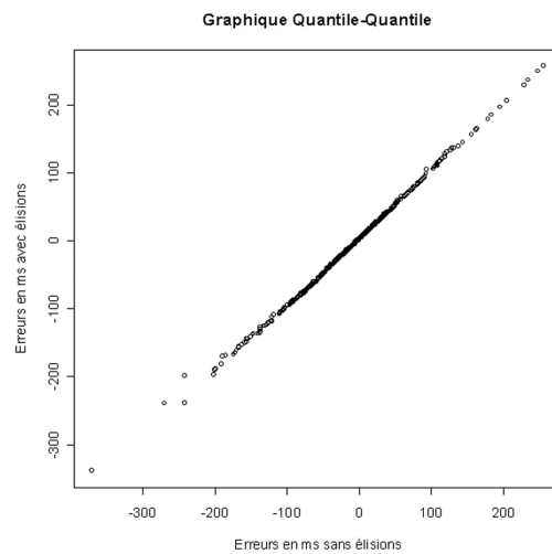
Figure 4 Graphique quantile-quantile des distributions des erreurs pour les alignements fondés sur les phonétisations sans et avec élisions
