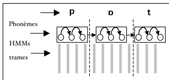
Figure 3 Attribution par l'algorithme Viterbi des trames temporelles aux états émetteurs des HMMs
