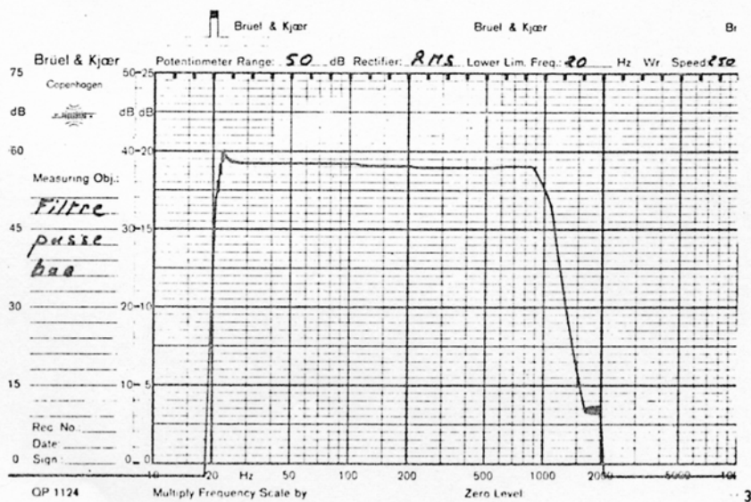
COURBE DE REPONSE DU DETECTEUR, DU FILTRE PASSE-HAUT ET DU FILTRE PASSE-BAS.
